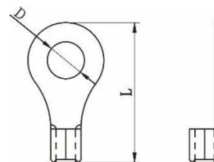
Кольцевой наконечник
