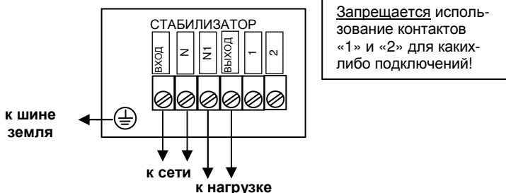
Рисунок 6.1 Схема подключения стабилизатора R4500C(K) (R6000C(K), R7500C(K), R10000C(K), R12000C(K))
